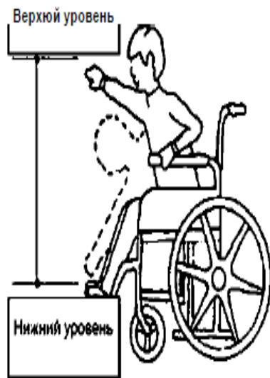
Зона легкодоступности вид сбоку
