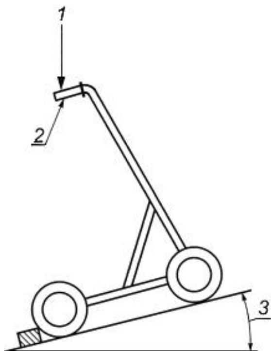
Рисунок 8 - Схема нагружения при испытании на заднюю устойчивость
