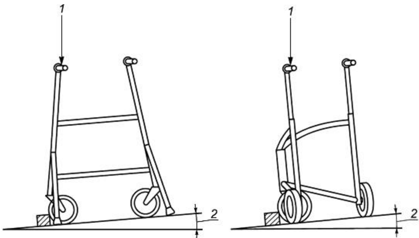
Рисунок 9 - Схема нагружения при испытании на боковую устойчивость
