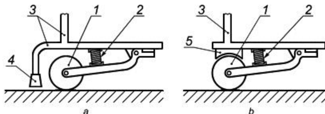
Рисунок 6 - Два технически различных вида прижимных тормозов
