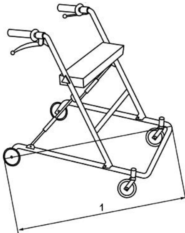
Рисунок 2 - Максимальные размеры ходунков
