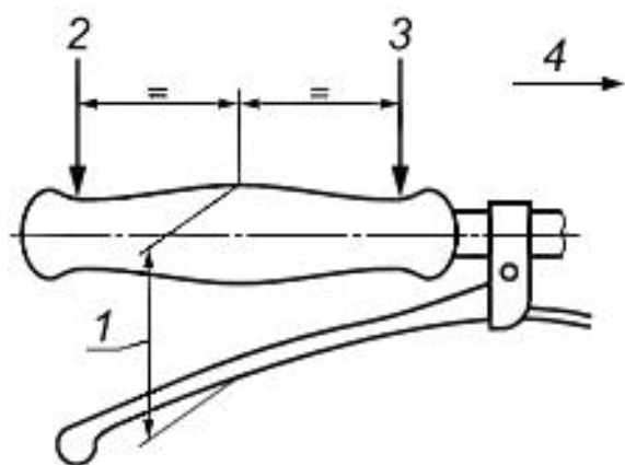
Рисунок 4 - Расстояние до рычага тормоза
