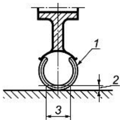
Рисунок 5 - Измерение ширины колесика
